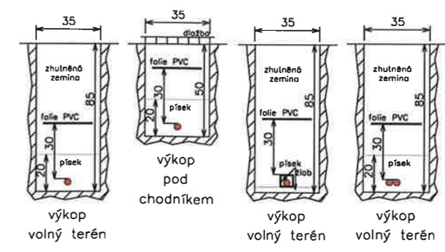
Řez uložením kabelu:
