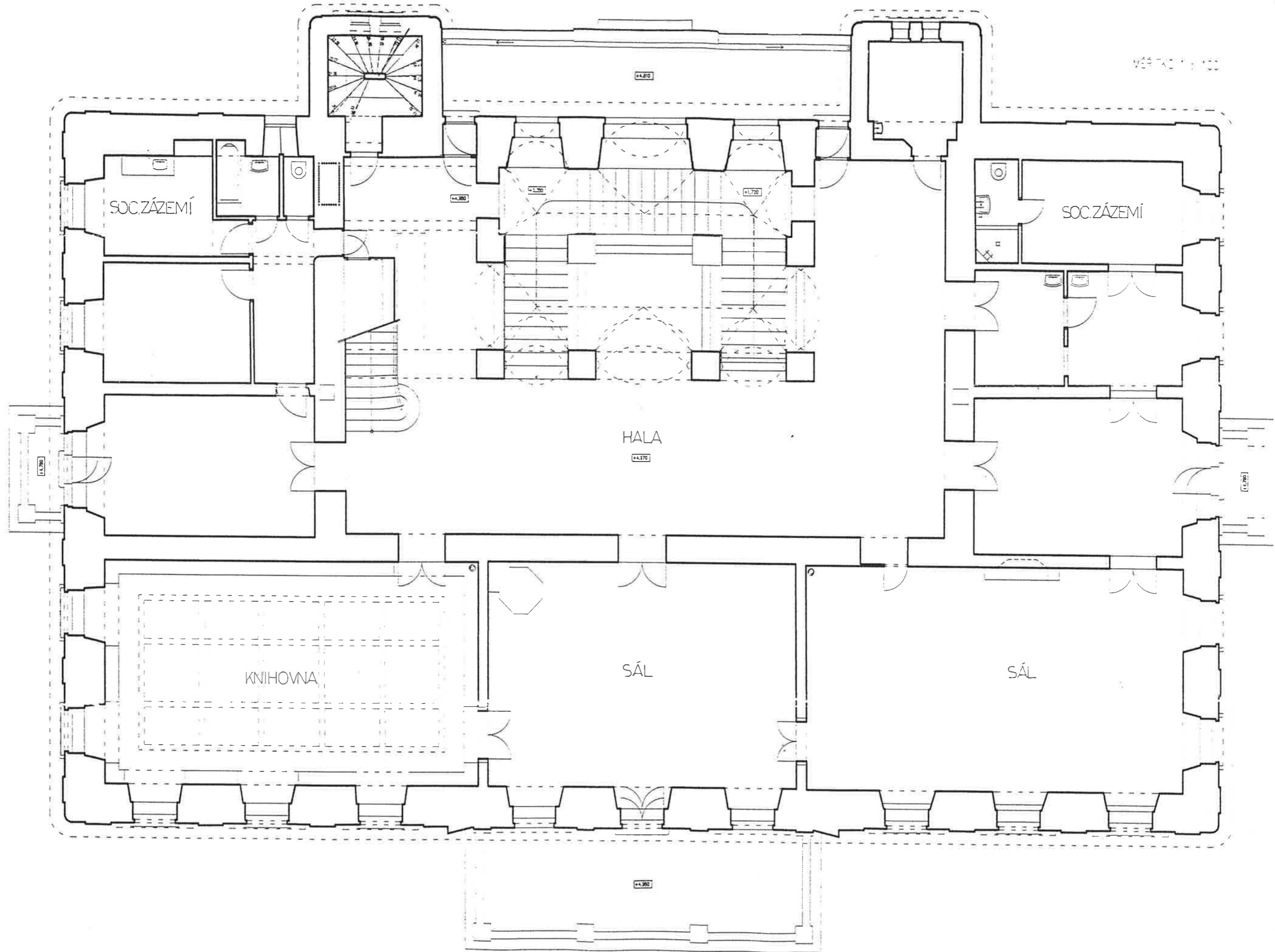
ZÁMEK - HROCHŮV TÝNEC Záměr využití 2., 3., a 4. nadzemního podlaží zámku Půdorys 2. NP – stav 1 : 100 výkres č. 1
